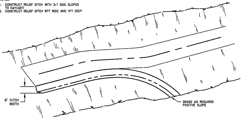
② RELIEF DITCH N.T.S.
