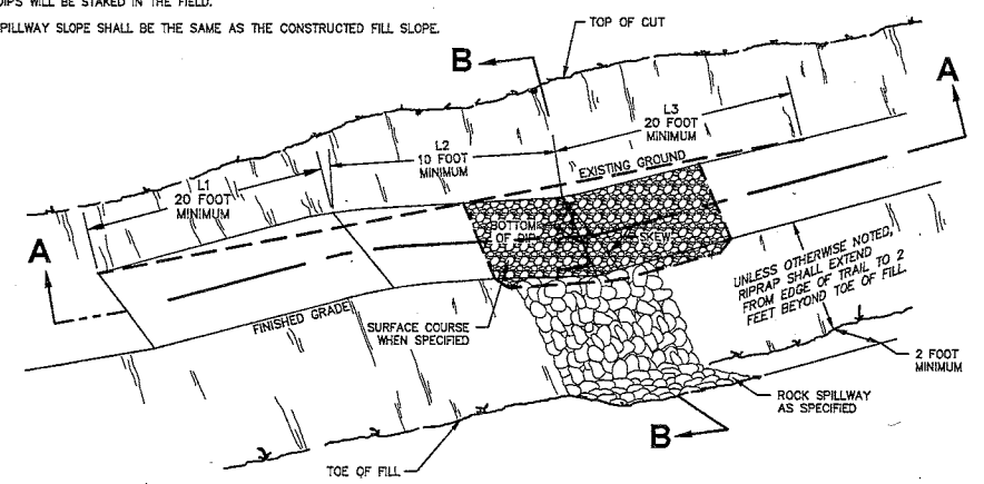
③ DIP DRAIN N.T.S.
